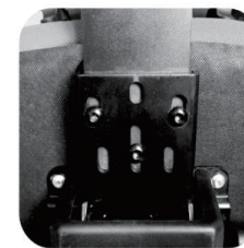
Схематичний приклад встановлення механізму крісла
