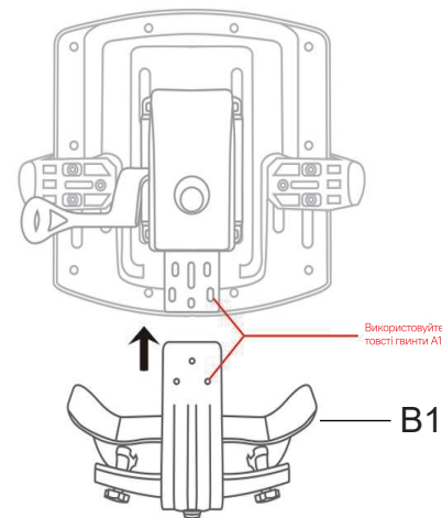
Схематичний приклад встановлення механізму крісла
